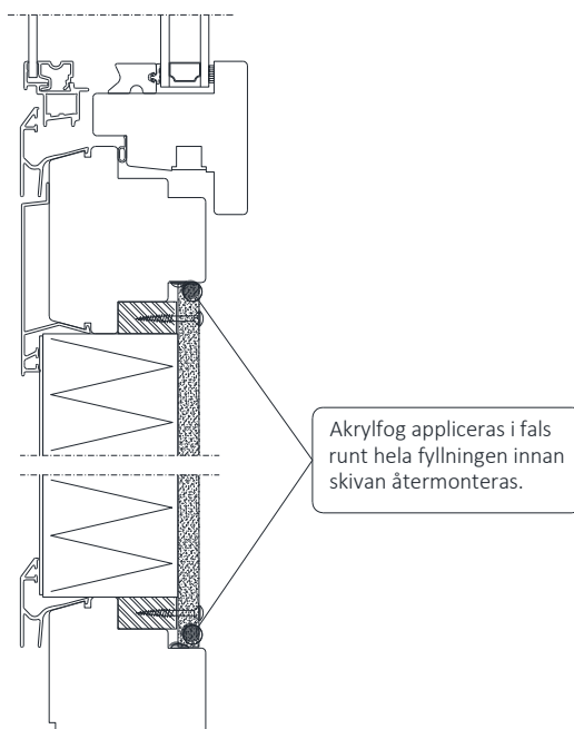
Vertikalsnitt
