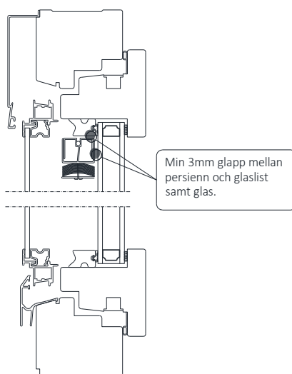
Vertikalsnitt
