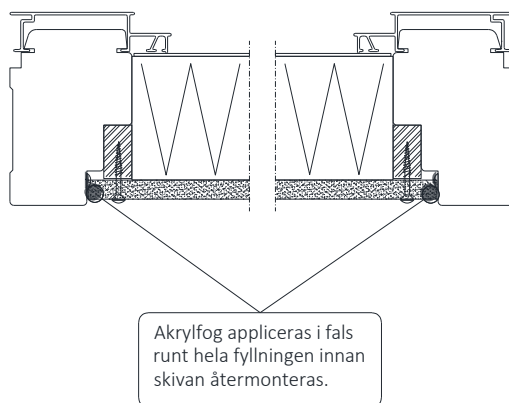
Horizontalsnitt
