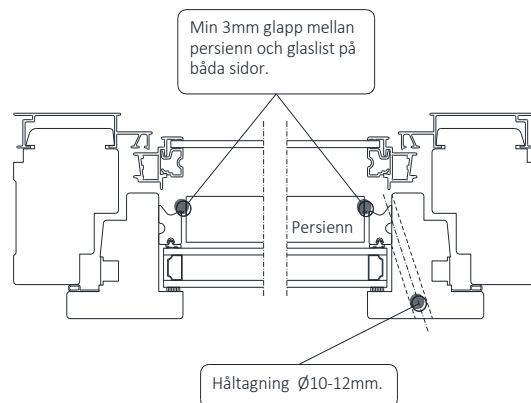
Horizontalsnitt
